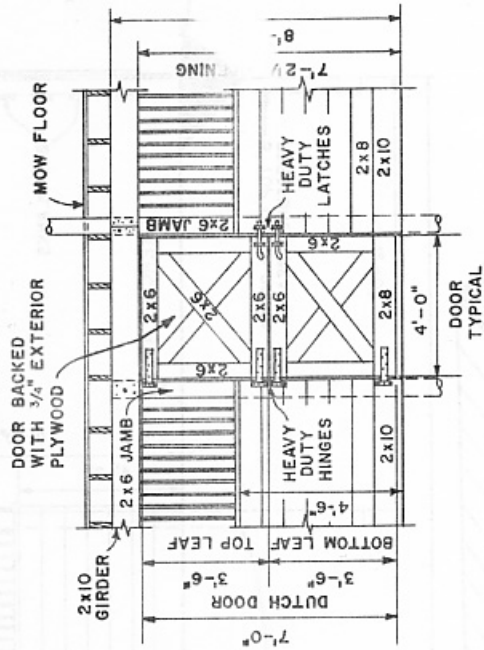
ELEVATION C-C
