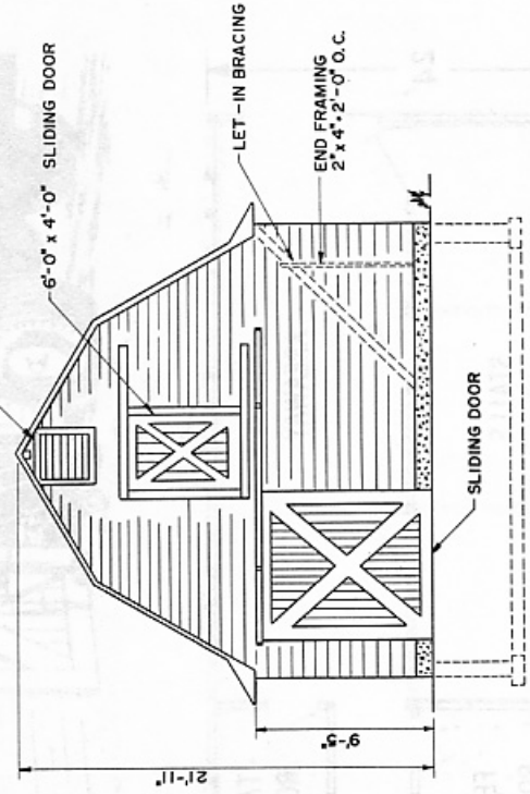
END ELEVATION
